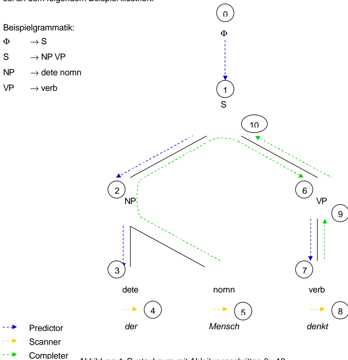
Abbildung 1: Syntaxbaum mit Ableitungsschritten 0 - 10
