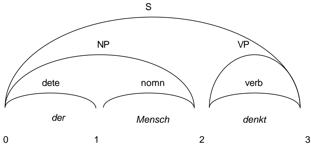
Abbildung 2: Kanten des Syntaxbaumes und ihre Abdeckung bezogen auf die Eingabe von der linken Grenze 0 (vor Wort 1) bis zur rechten Grenze 3 (hinter Wort 3)
